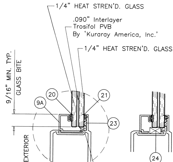
DOOR LEAF GLASS TYPE 'A'
