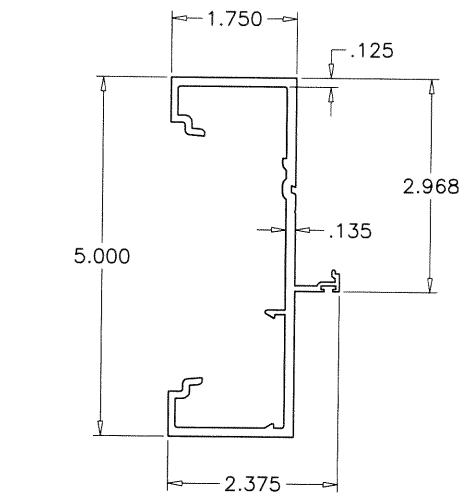
2 DOOR FRAME JAMB
