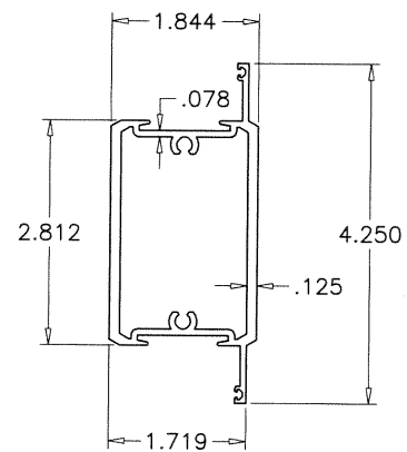
12 INTERMEDIATE HORIZ.
