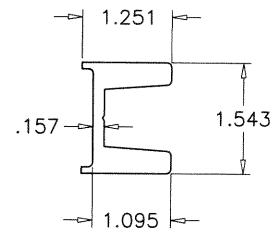
14 ASTRAGAL STIFFENER
